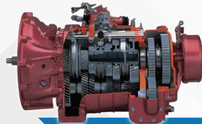
7前速超速檔鋁合金波箱
