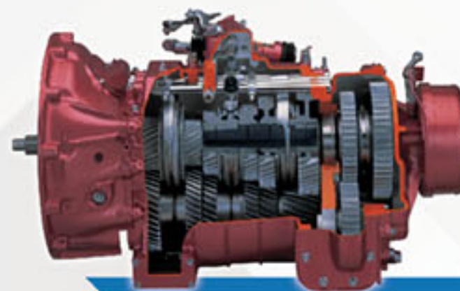
7前速超速檔鋁合金波箱 採用先進同步器，操作容易，入波暢順。
